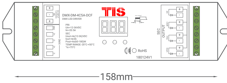
▲ DMX Sürücünün Boyutları
