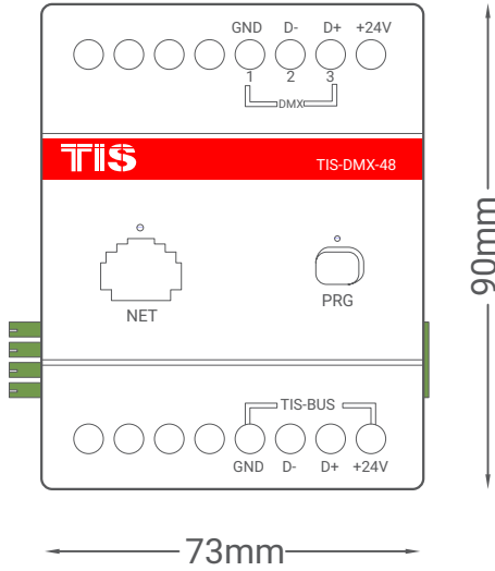
▲ TIS-DMX-48 Modül Boyutları
