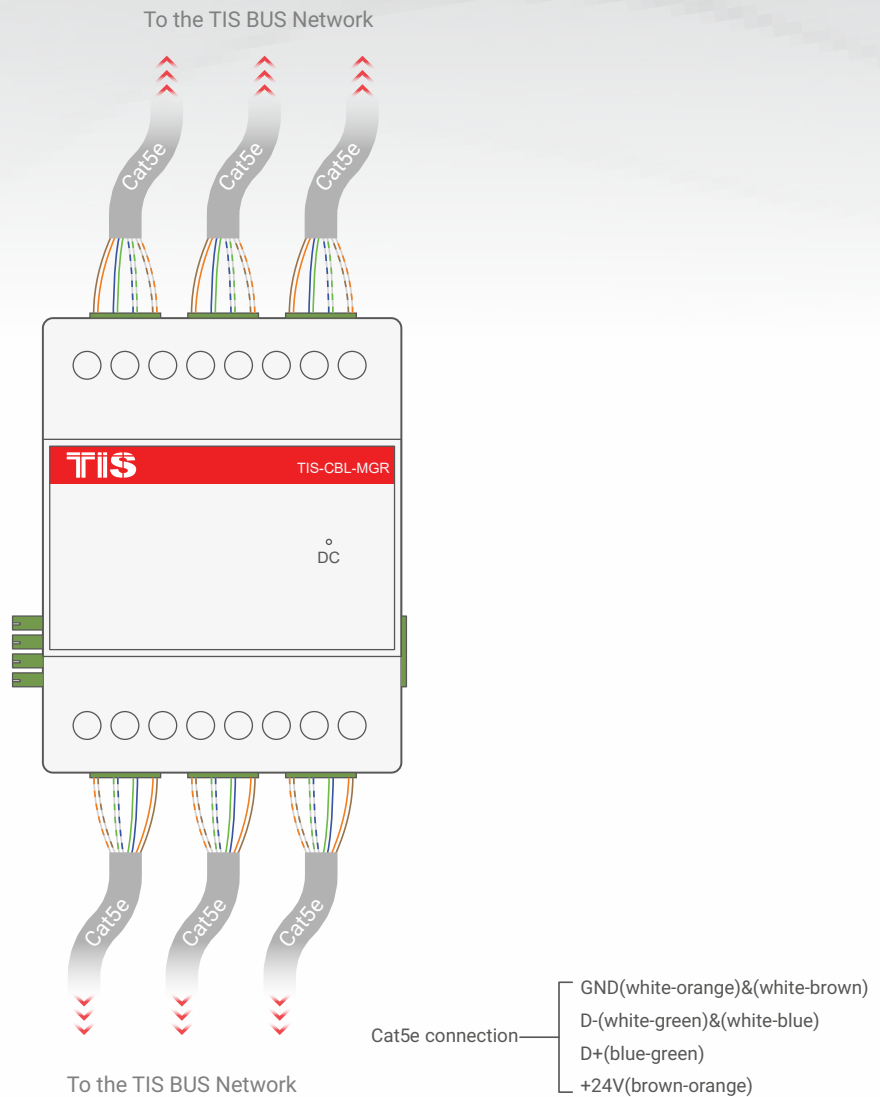
▲ Modül BUS Bağlantı Şekli
