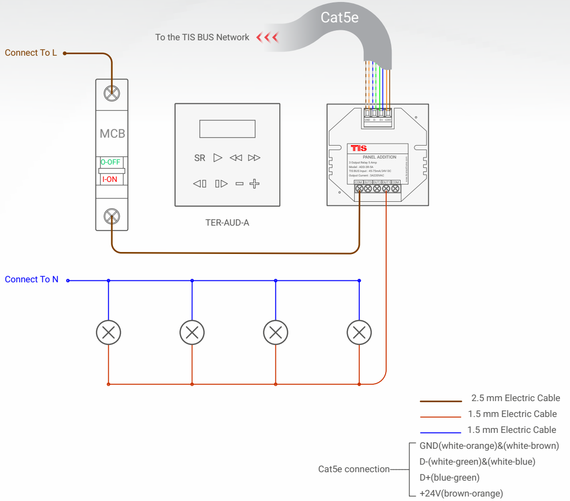
▲ TER-AUD-A ve ADD-3R-5A Aydınlatma Bağlantı Diyagramı
