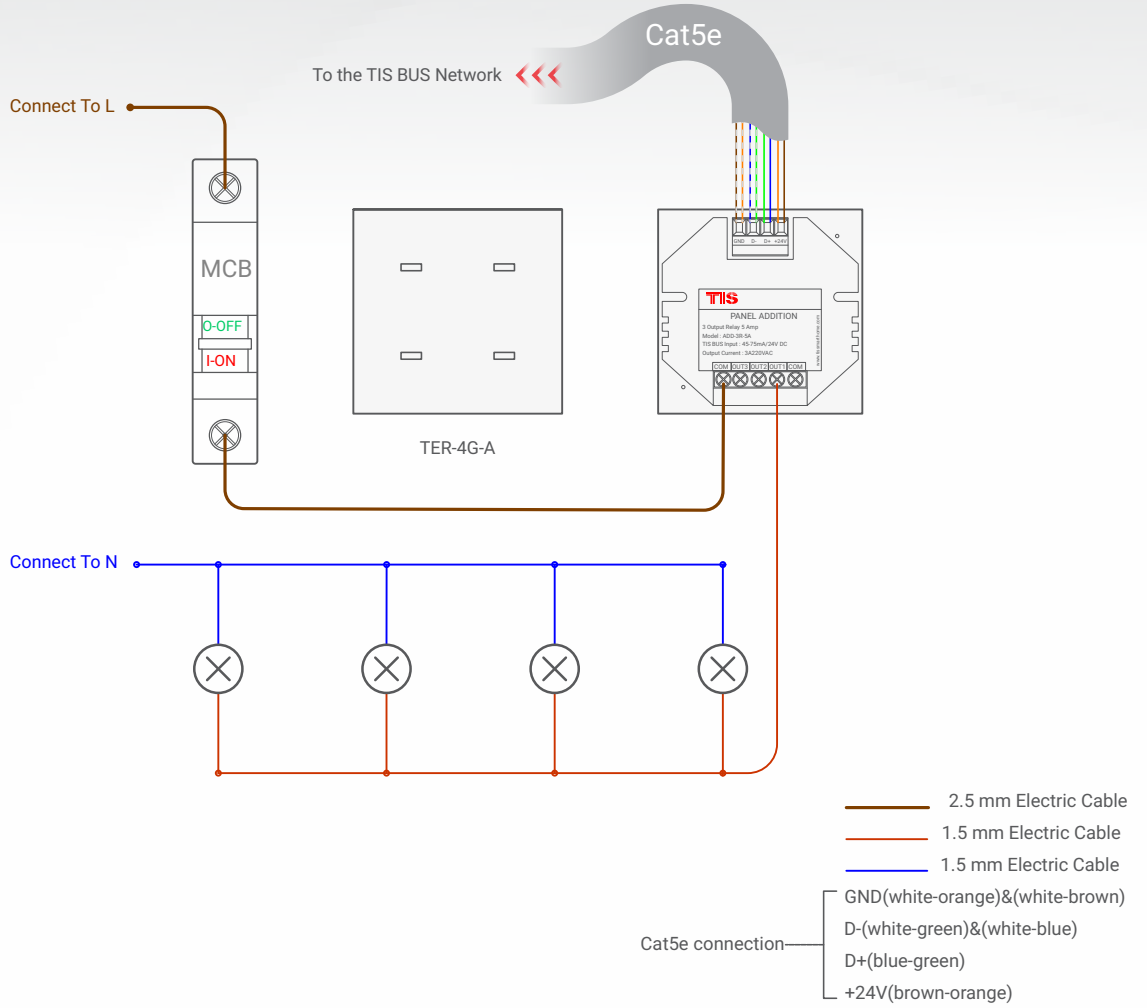
▲ TER-4G-A & ADD-3R-5A Aydınlatma Bağlantı Diyagramı
