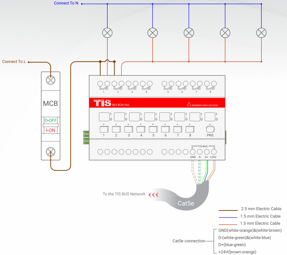
▲ Aydınlatma Bağlantı Diyagramı
