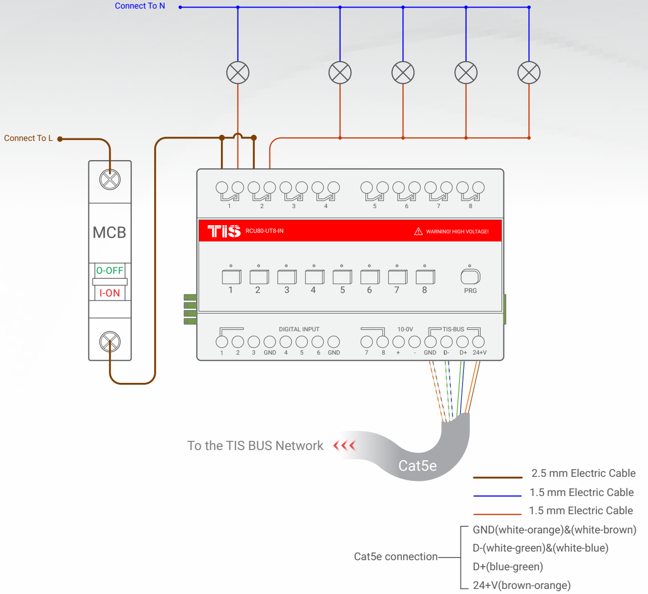
▲ Aydınlatma Bağlantı Diyagramı
