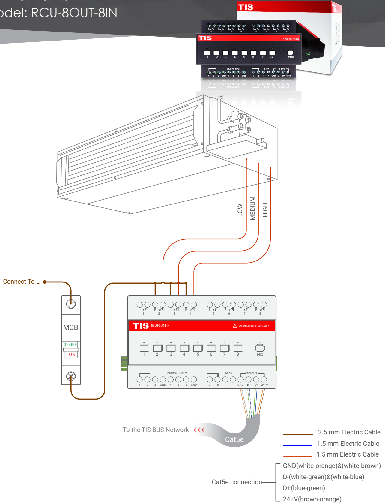
▲ Figure 1: FCU Bağlantı Diyagramı
