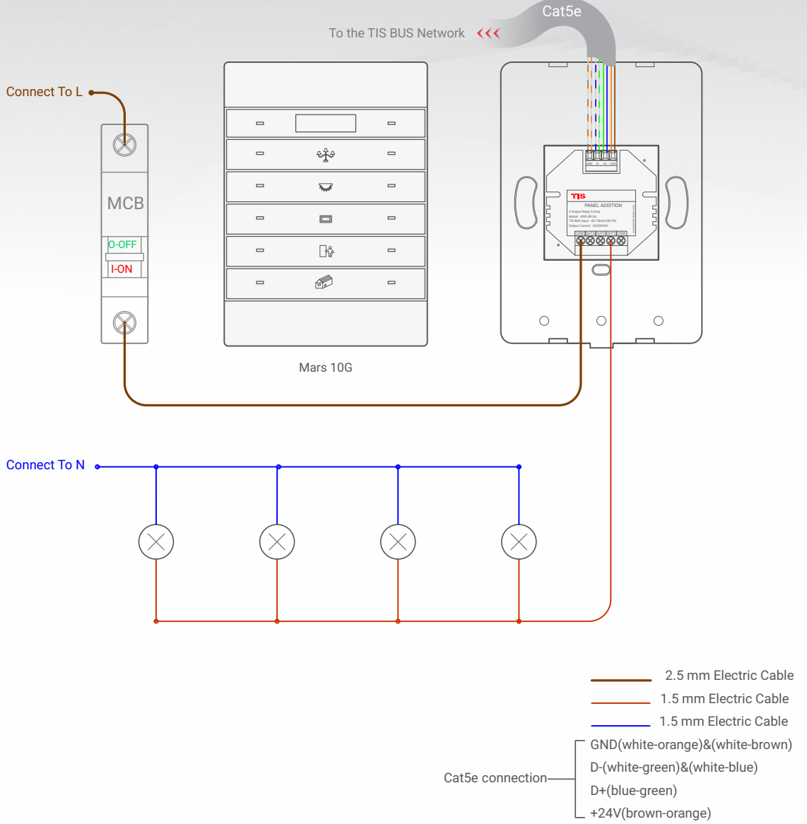
▲ Mars 10G & ADD-3R-5A Aydınlatma Bağlantı Diyagramı
