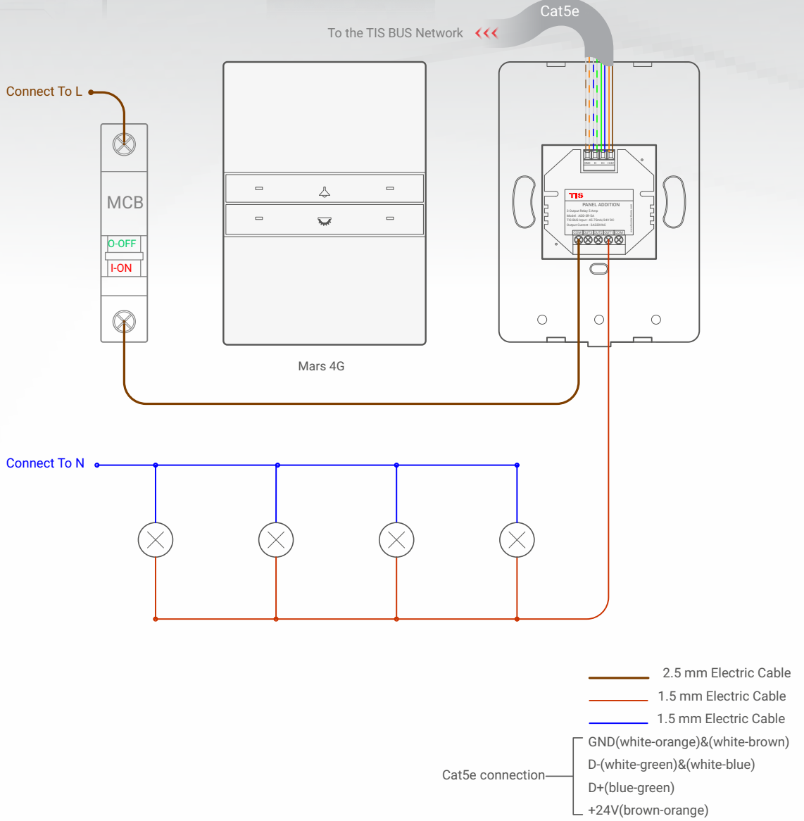
▲ Mars 4G ve ADD-3R-5A Aydınlatma Bağlantı Diyagramı
