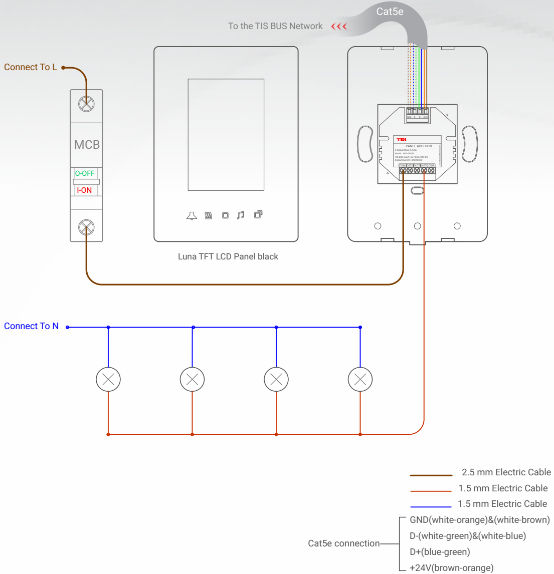
▲ Luna TFT ve ADD-3R-5A Aydınlatma Bağlantı Diyagramı
