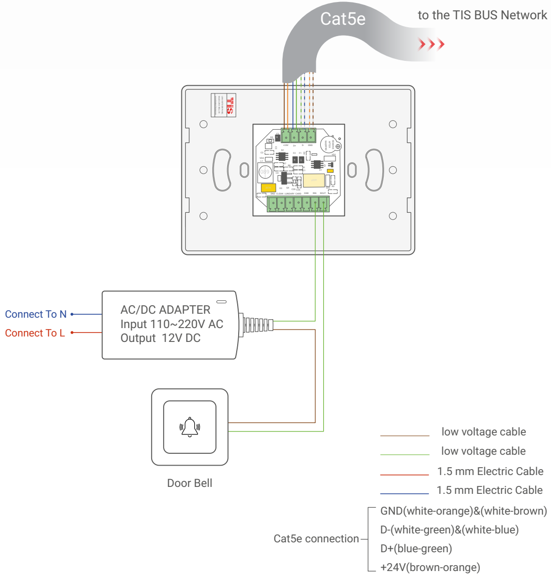
▲ LUNA-BELL-3S ve Kapı Zili Birimi Bağlantı Diyagramı
