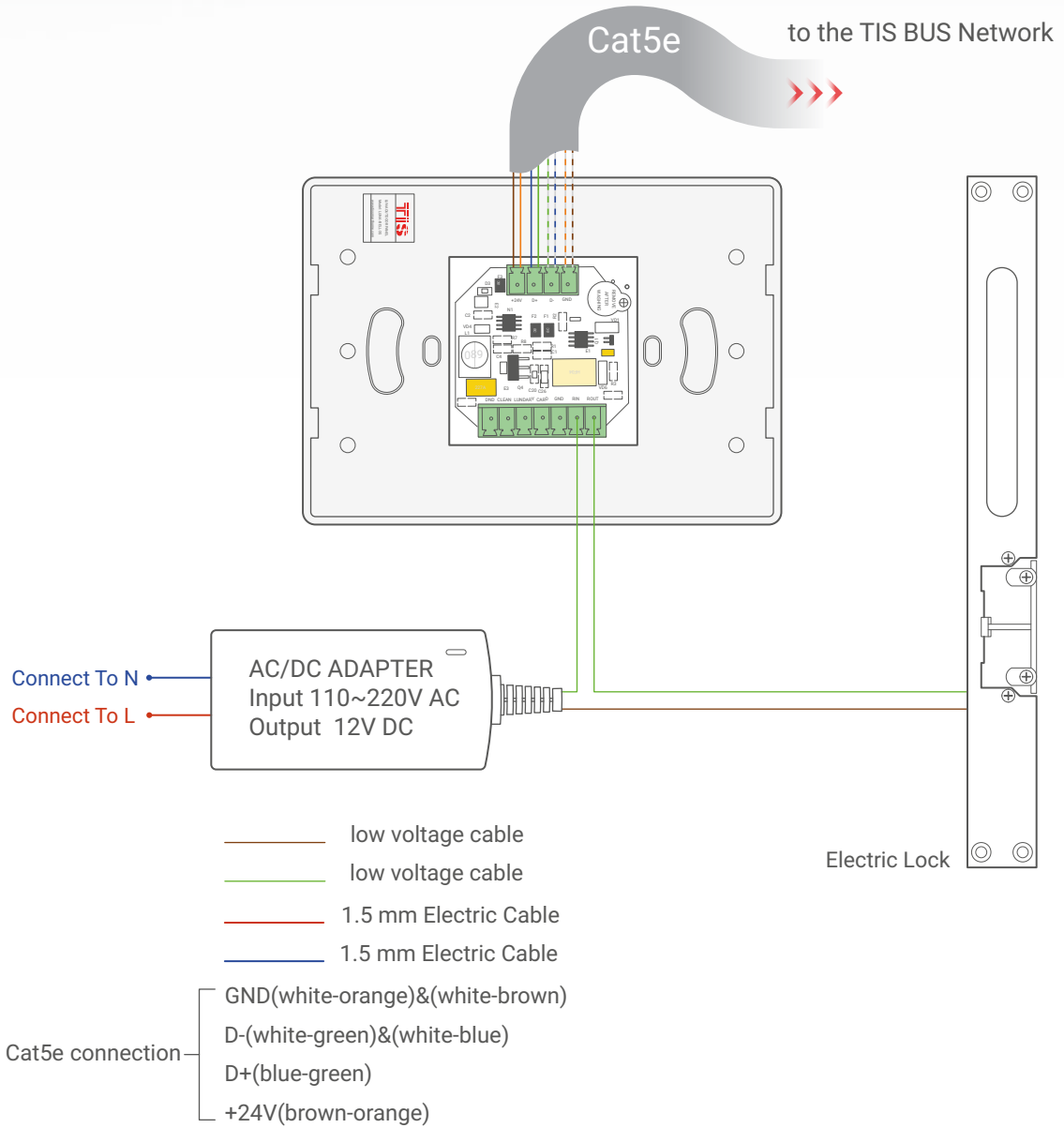
▲ LUNA-BELL-3S-RF ve Elektrik Kilidi Bağlantı Diyagramı
