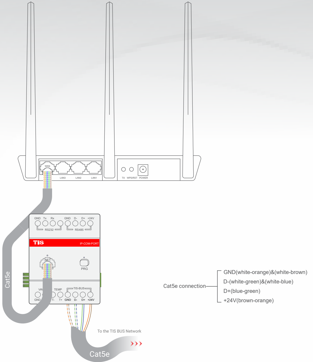
▲ IP Ağ Geçidi ve Modem Bağlantı Diyagramı
