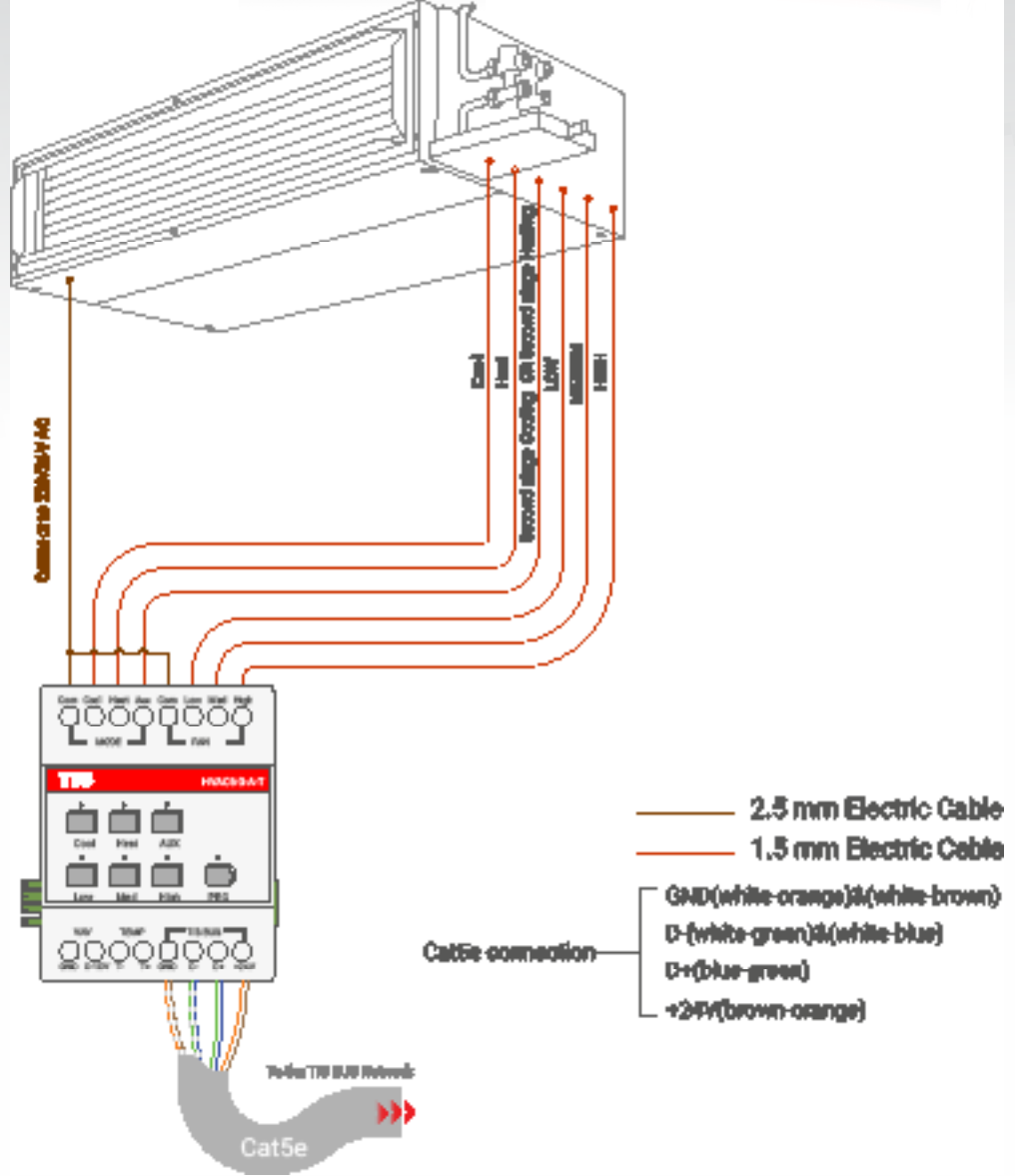
▲ FCU Bağlantı Diyagramı
