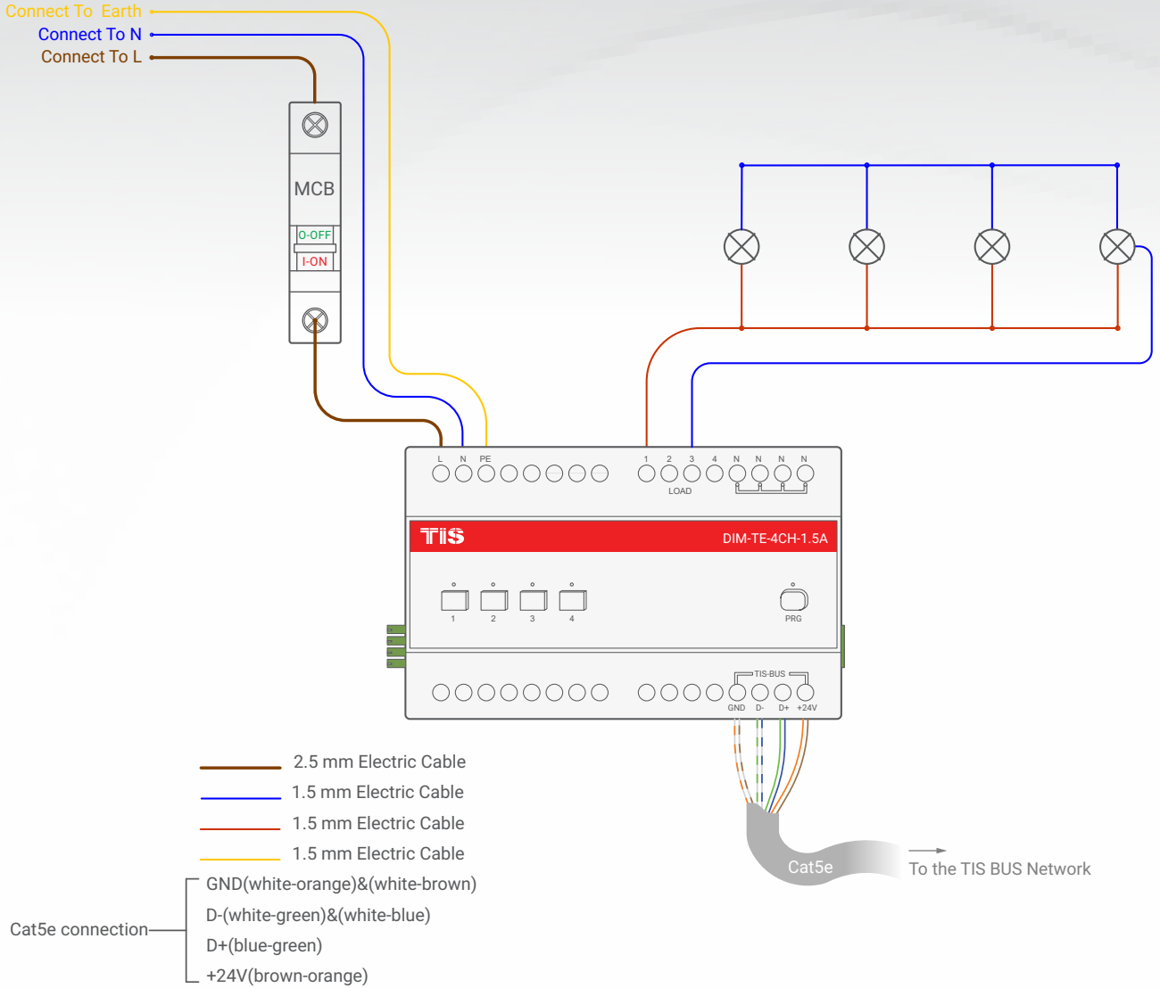
▲ Aydınlatma Bağlantı Diyagramı
