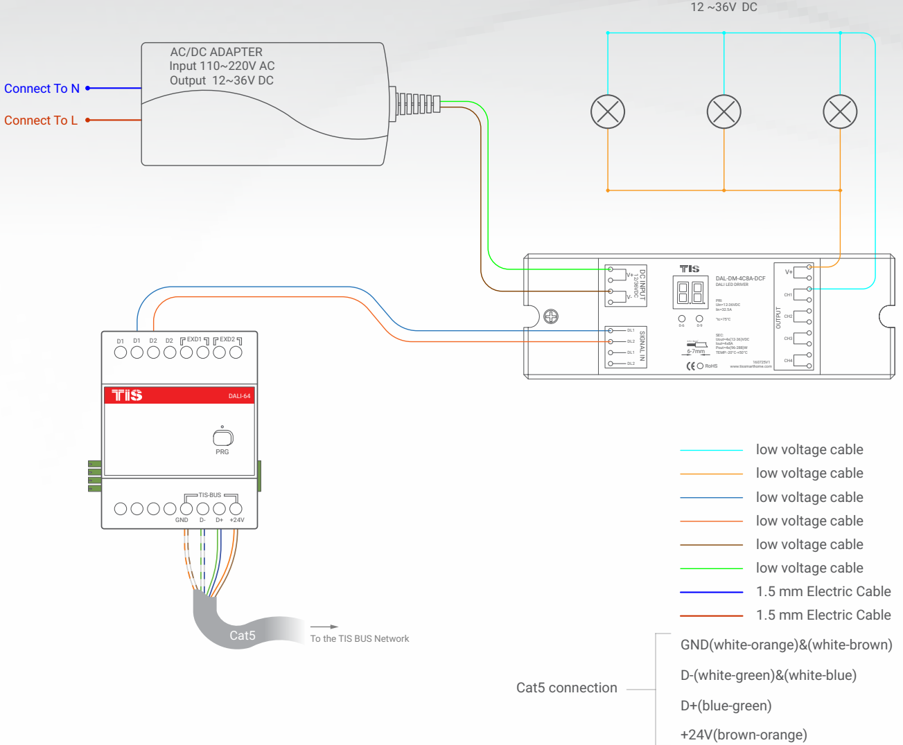
▲ Dalı Sürücü ve Aydınlatma Bağlantı Diyagramı
