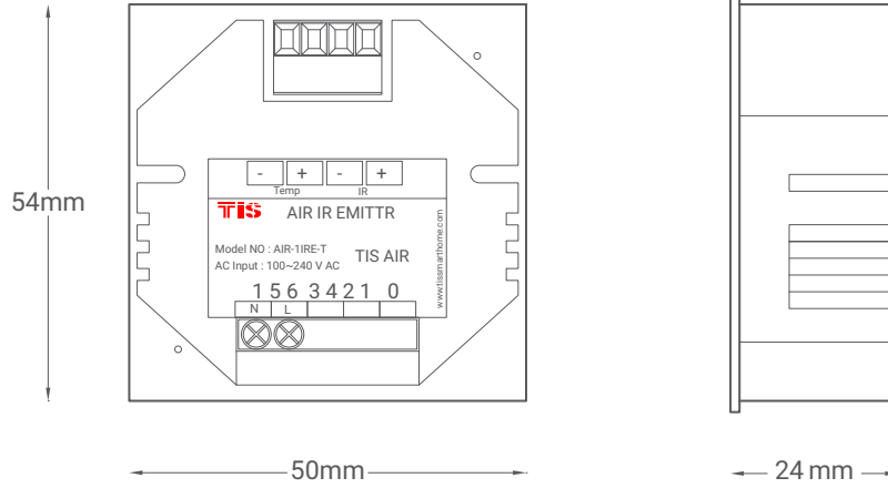
▲ Modül Boyutları
