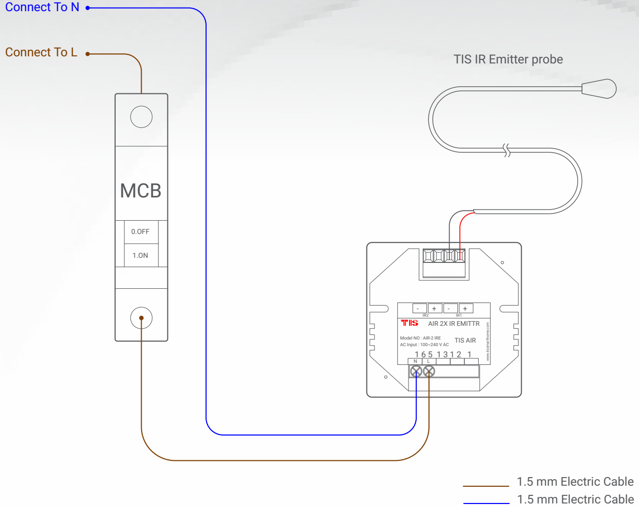
▲ LED Dimmer Bağlantı Diyagramı
