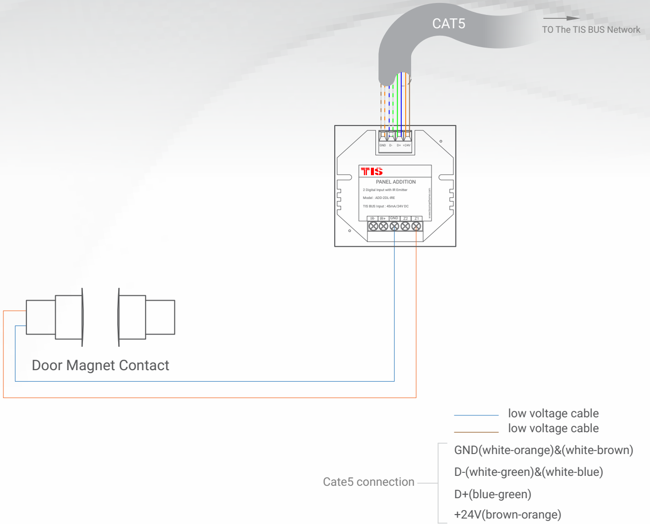
▲ ADD-2DL-IRR ve Manyetik Kontak Bağlantı Diyagramı
