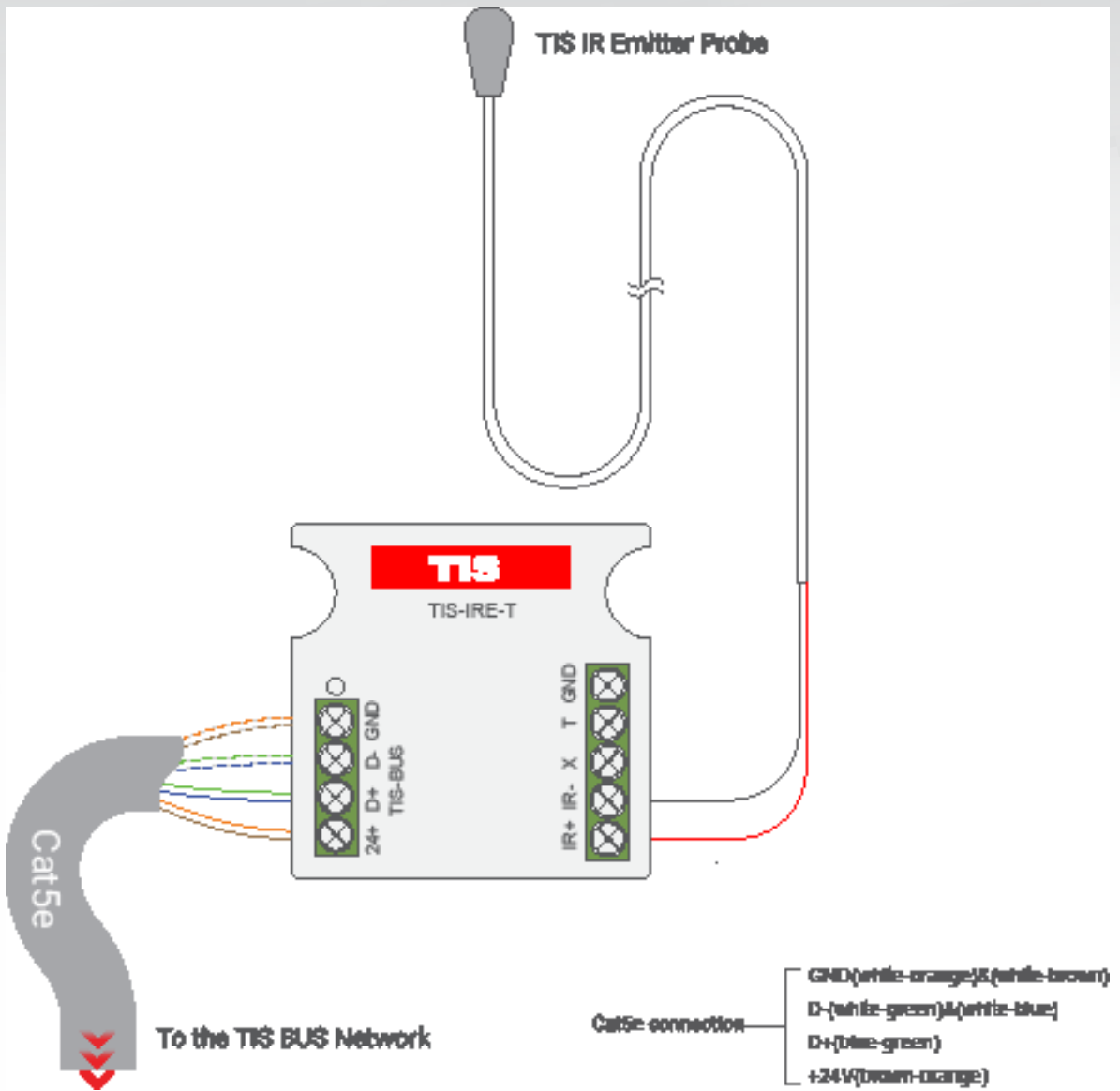
▲ TIS Kızılötesi Verici Göz Bağlantı Diyagramı
